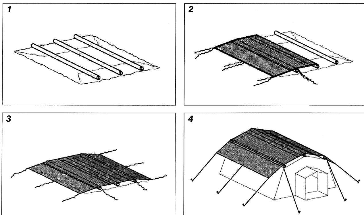
Figura 2.12 – Sequenza di montaggio del telo ombreggiatore.
