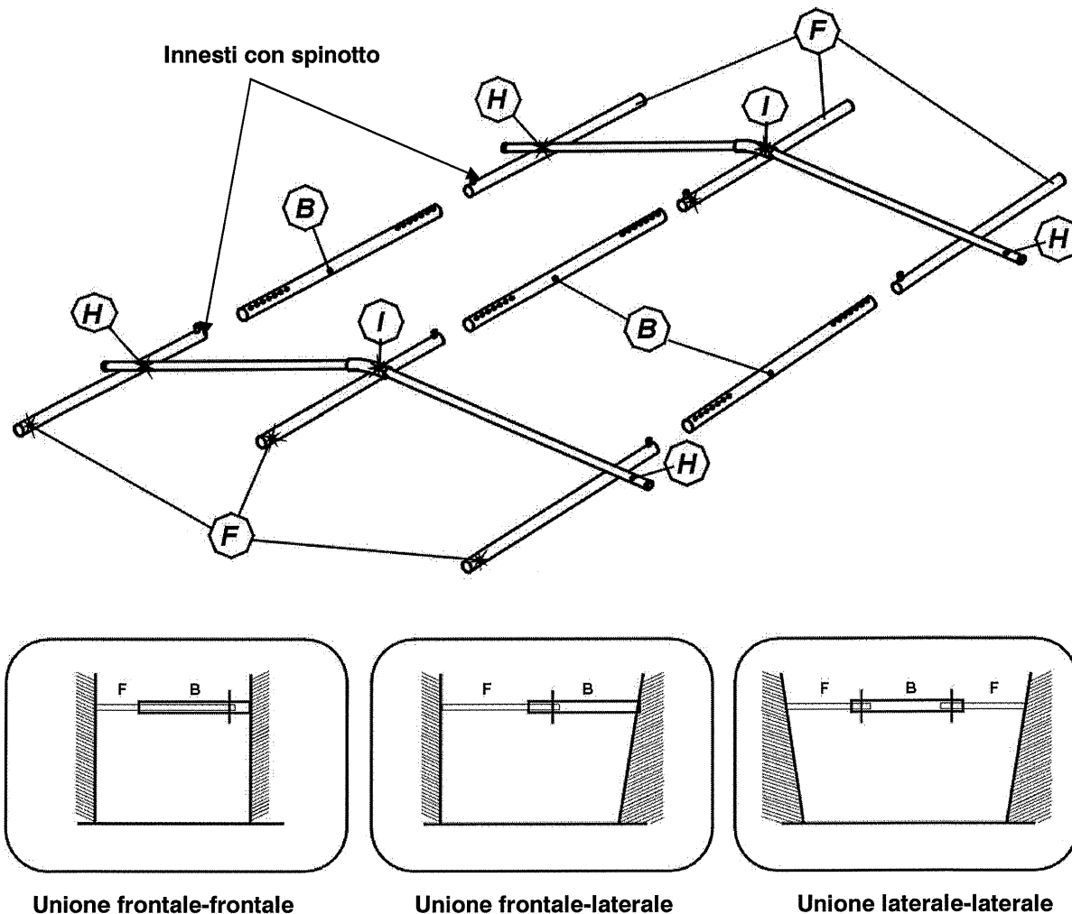
Figura 2.19 - Schema di montaggio della paleria per corridoio di unione tende
