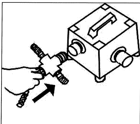
Figura 3.1 - Innesto della tubazione al gonfiatore per aspirazione.
