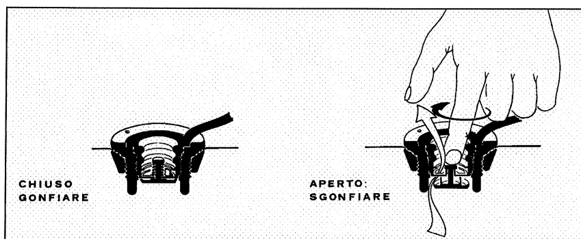
Figura 2.2 – Chiusura delle valvole di gonfiaggio.
