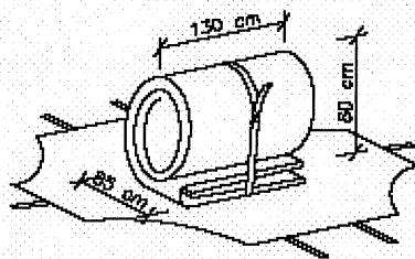
Figura 3.8 – Posizionamento nel sacco.
