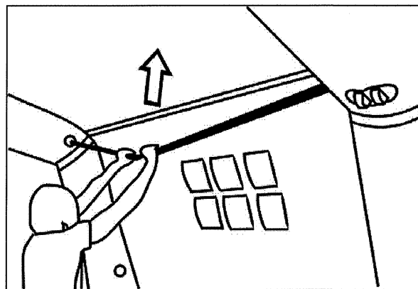
Figura 2.7 - Montaggio aste distanziali.
