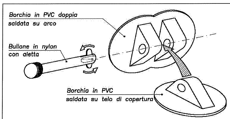
Figura 5.2 - Connessione mediante bullone con aletta.
