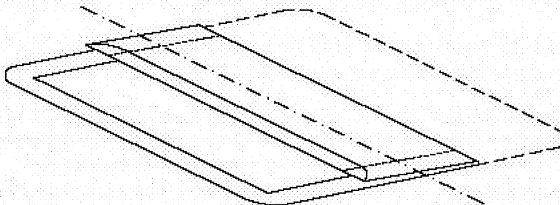
Figura 3.4 – Prima piega (lato dx).
