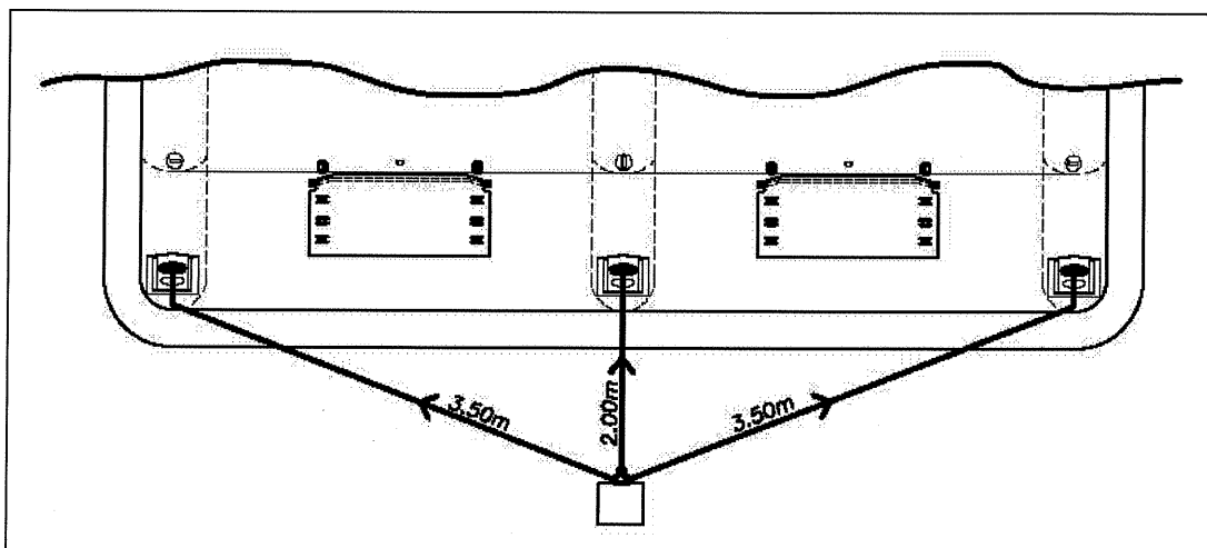
Figura 2.3 – Schema del Kit gonfiaggio simultaneo.
