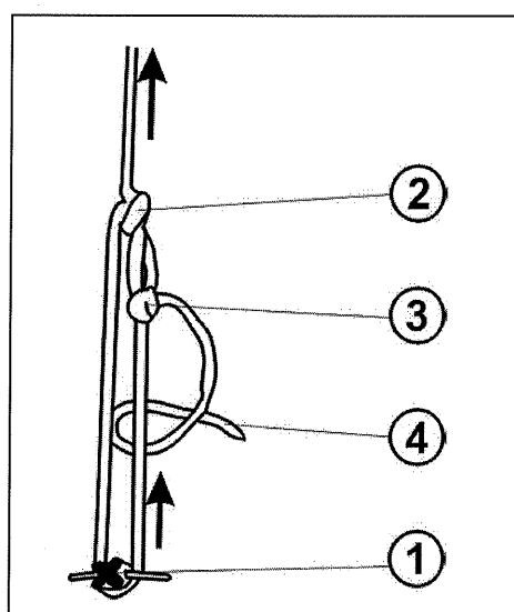
Figura 2.14 – Schema di realizzazione del cappio e nodo sul tirante.
