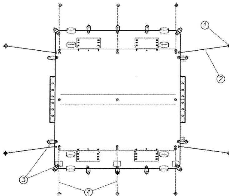
Figure 2.8 – Distanziale installato.
